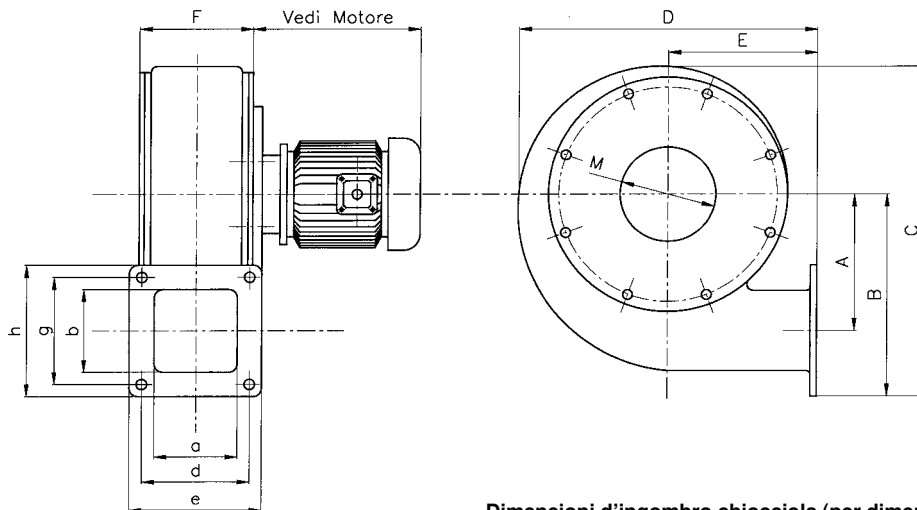
Dimensioni d'ingombro chiocciola (per dimensioni motore vedi pag. 298) Dimension of thread (for dimension of motors, see page 298) Platzbedarf spiralgehäuse (für motorabmessungen siehe seite 298) Encombrement carcasse (voir page 298 pour les dimensions moteur) Dimensiones exteriores de la carcasa (para las dimensiones del motor véase la página 298)
